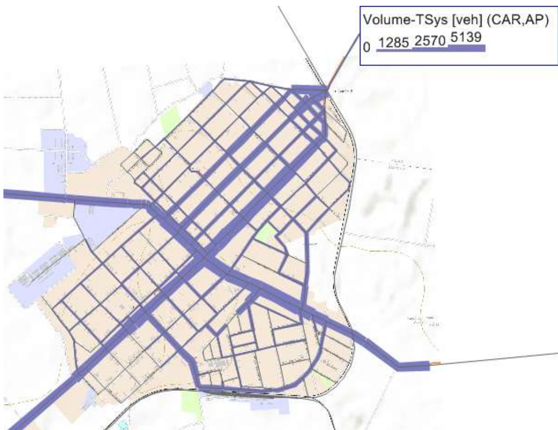
Figura 3.6-2 Mărimea fluxurilor rutiere de trafic – prognoză 2033
